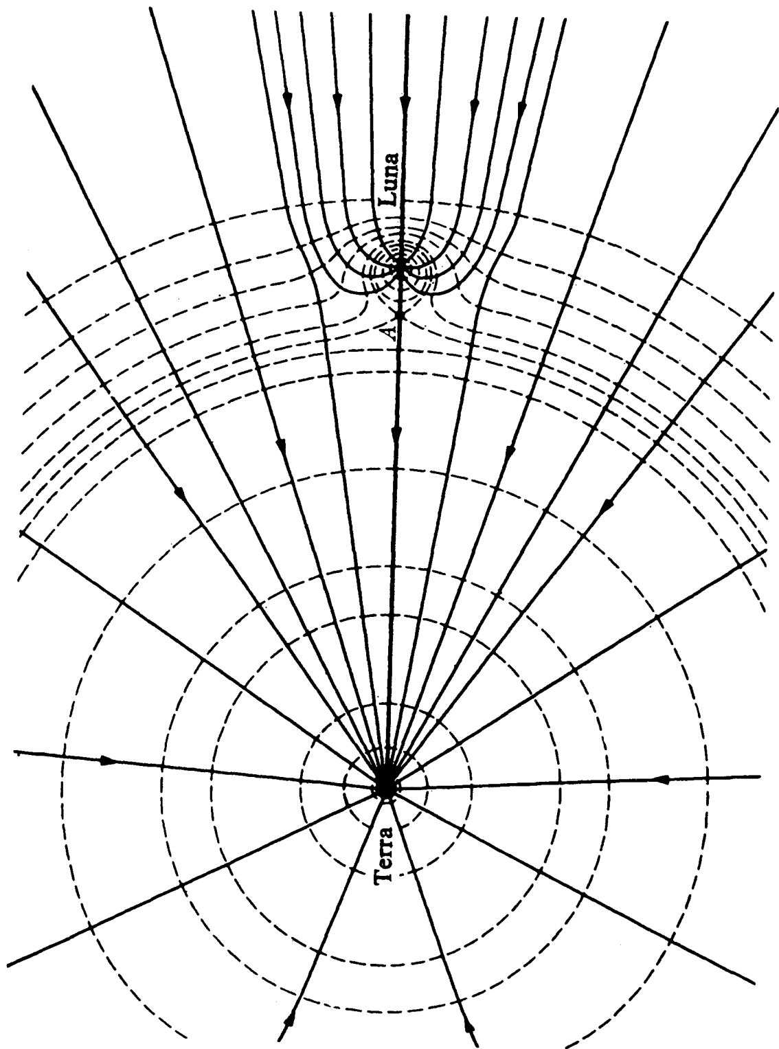
Fig. 13-17. Linee di forza e superfici equipotenziali del campo gravitazionale prodotto dalla terra e dalla luna. In A il campo gravitazionale risultante è nullo. [Da W. T. Scott, Am. J. Phys. , 33 , 712 (1965)]
